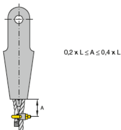
Serre-câble selon la norme EN 13411-5
